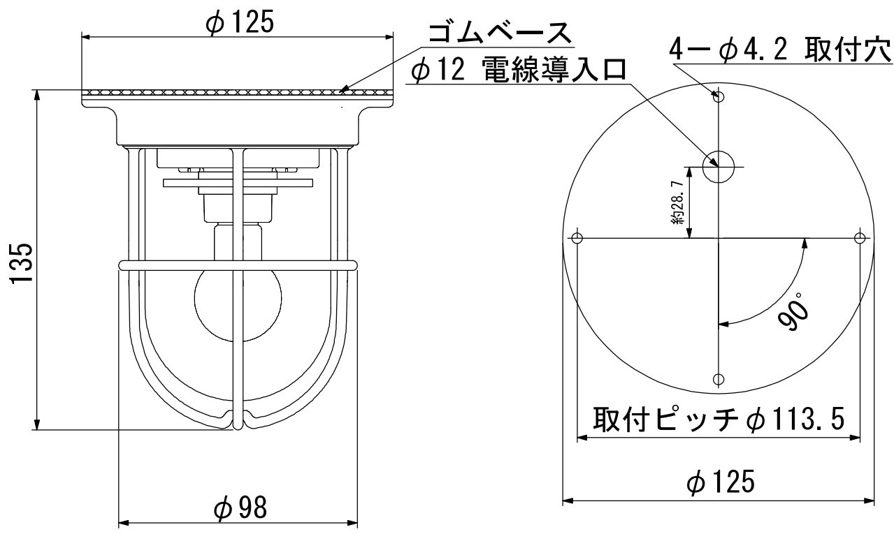
<<取付面 寸法図>>
