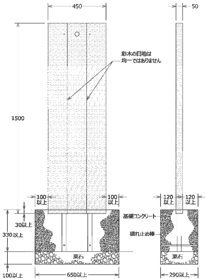
【正面図】
