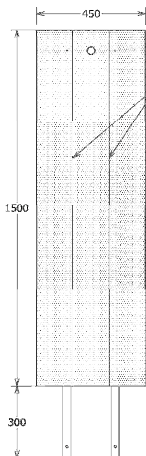
【正面図】
