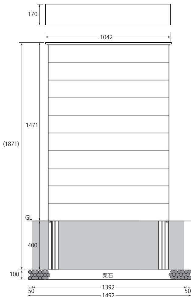
〔正面図〕
